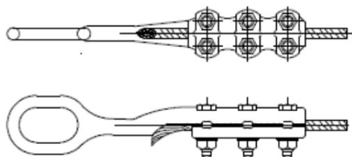
Fig. U MORSETTO DI AMARRO PER FUNE METALLICA MOORING CLAMP FOR WIRE ROPE
